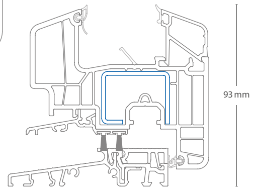
Bezbariérový práh balkonových dveří výška 20 mm / Obr.: 1:2
